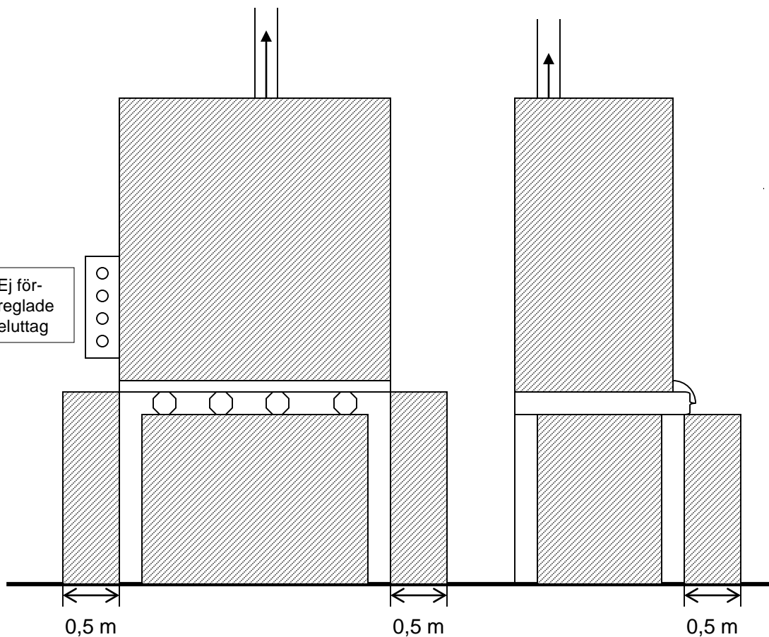
Dragskåp framifrån
